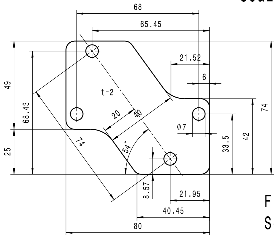
Front view Scale: 1:1
