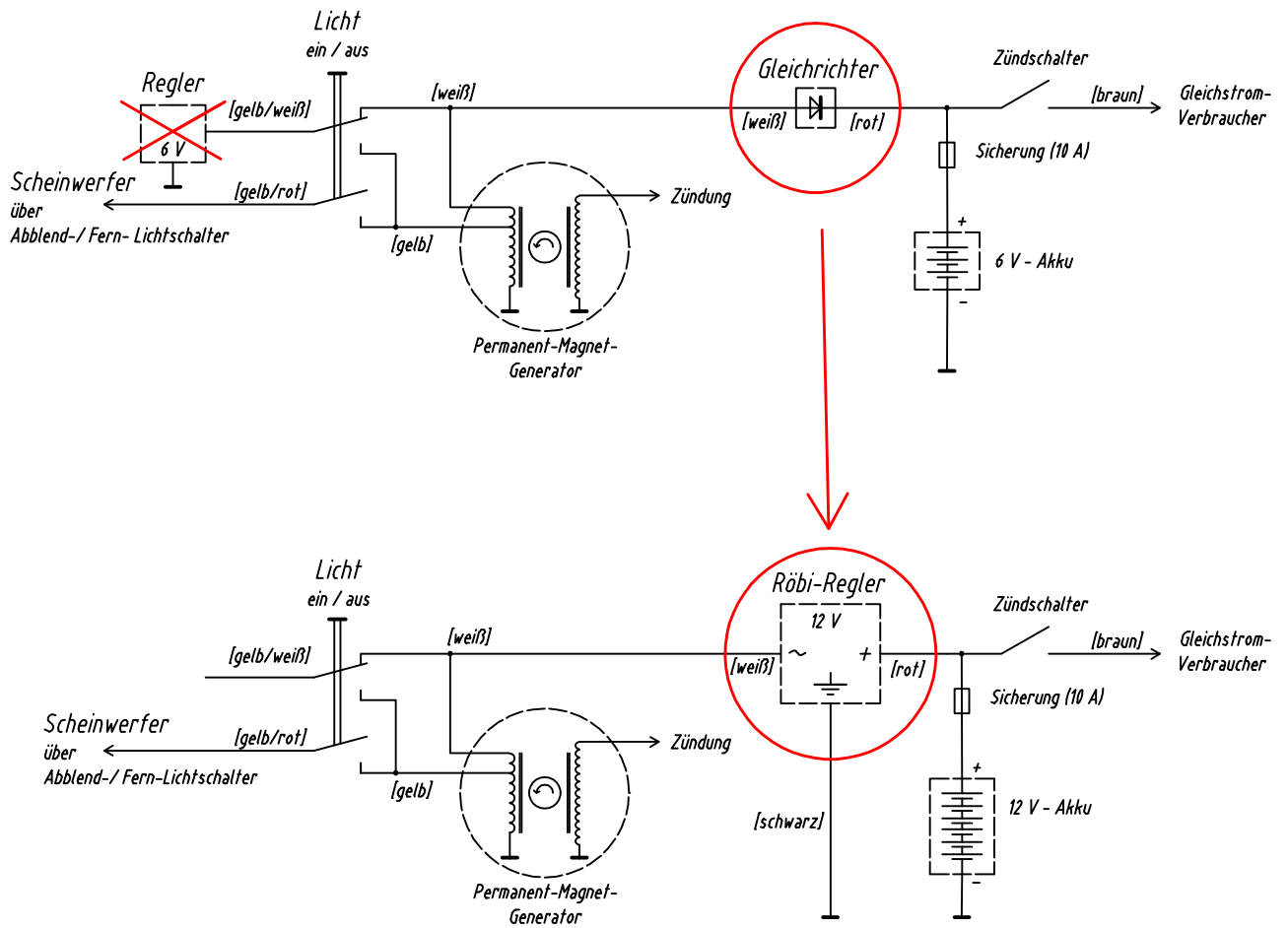
Umbau: Original 6 V-Elektrik -> 12 V-Röbi-Regler Kabelfarben [ ..... ] gültig für XT 500
